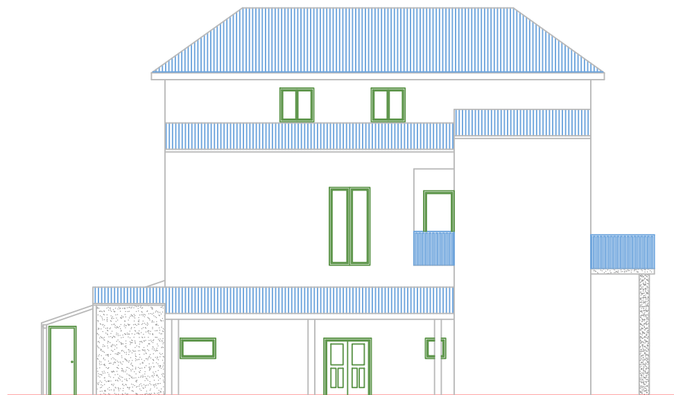
SJEVEROZAPADNO PROČELJE
