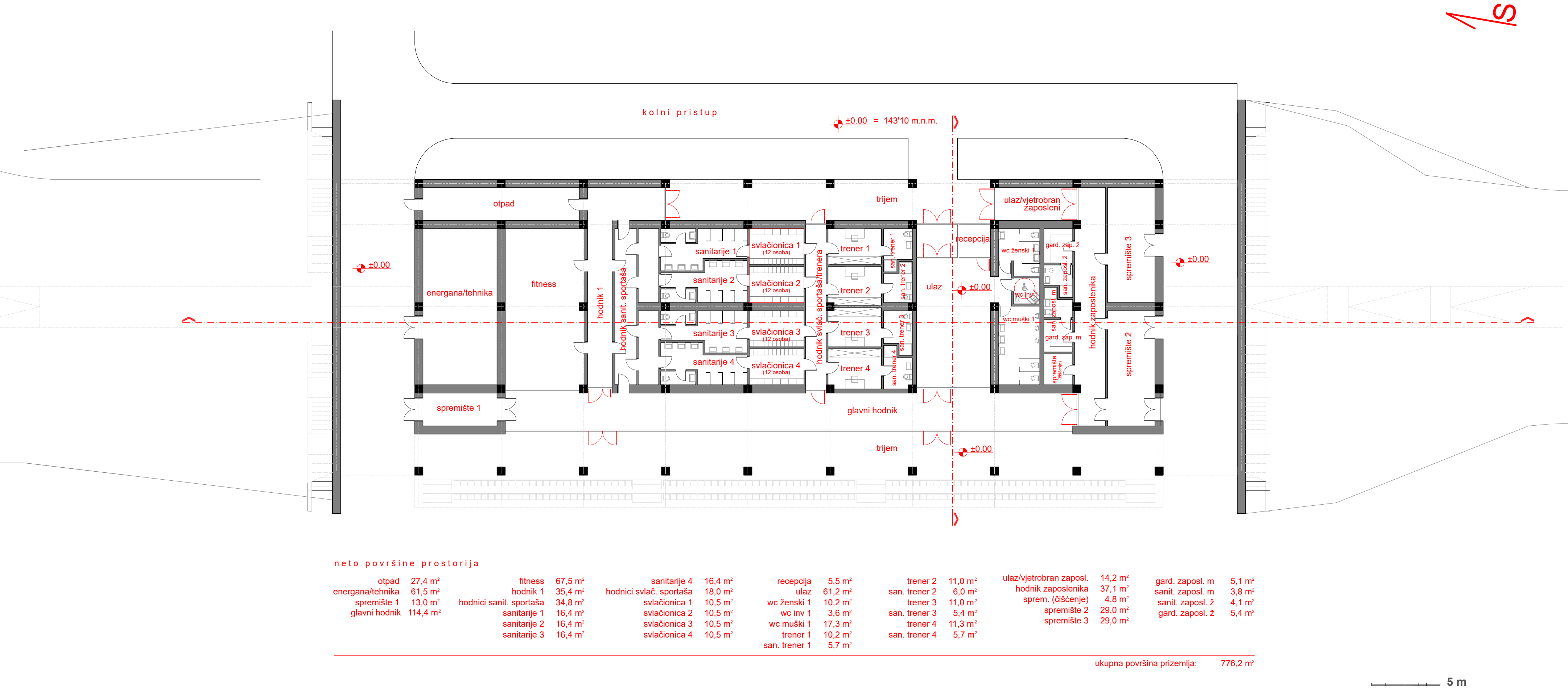
IDEJNO RJEŠENJE ZGRADE ATLETSKOG STADIONA POŽEGA TLOCRT PRIZEMLJA MJ 1:200 LIST 2
